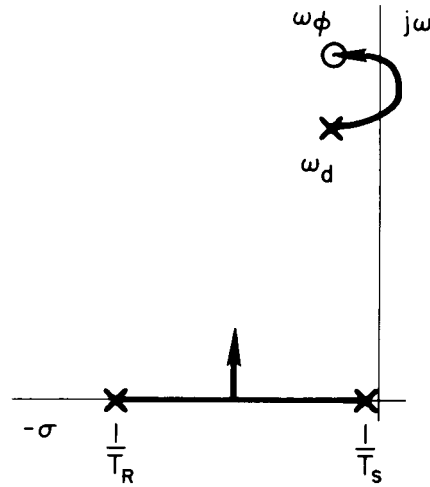
b) Low \zeta_d ; Zero Above Pole
