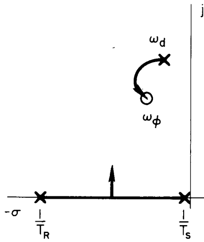
a) Low \zeta_d ; Zero Below Pole
